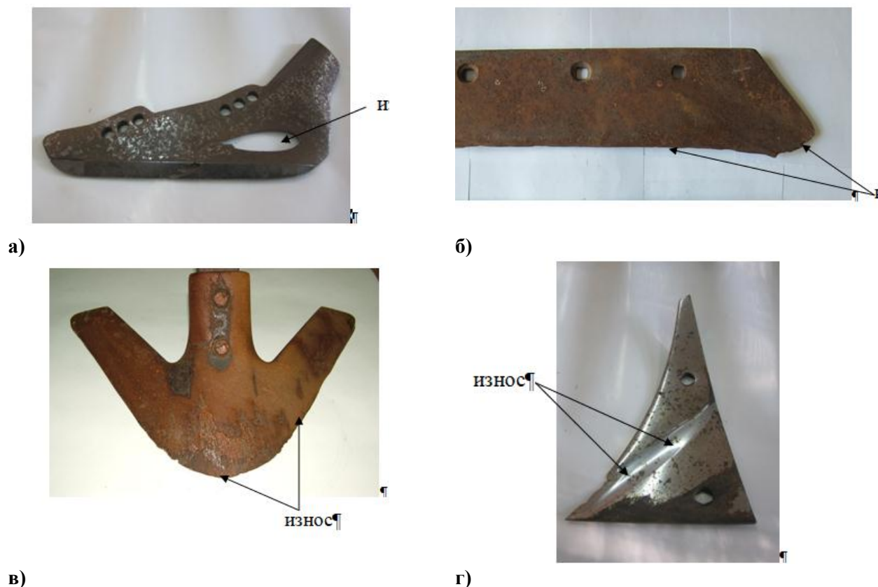
Рисунок 1 – Изношенные рабочие органы сельскохозяйственной техники: лемех свеклоуборочного комбайна ROPA Euro Tiger III (а); лемех плуга ПЛН-5-35 (б); стрелчатая лапа культиватора КПИ-4,2 (в); грудинка отвала плуга фирмы KUNN (г)
