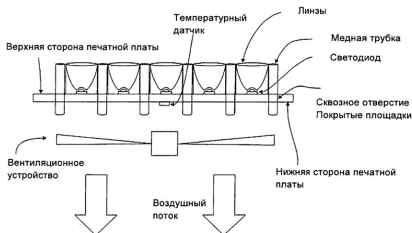
Рисунок 5 – Полупроводниковое устройство
